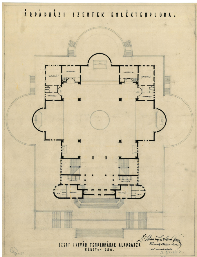
24. ábra. Kismarty-Lechner Jenő: Árpád-házi szentek templomának terve (Forrás: BTM Kiscelli Múzeum Építészeti Gyűjtemény no. 66.62.2.)
