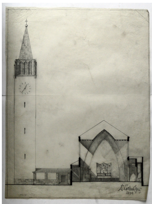
15. ábra. Kismarty-Lechner Jenő: A jelű tervvariáns az albertfalvai templomhoz (Forrás: BME Építészettörténeti Rajztár no. 101607)
